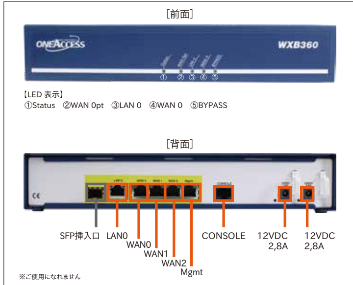
WAN 最適化・高速化装置 WXB360
