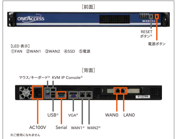
WAN 最適化・高速化装置 WXB550
