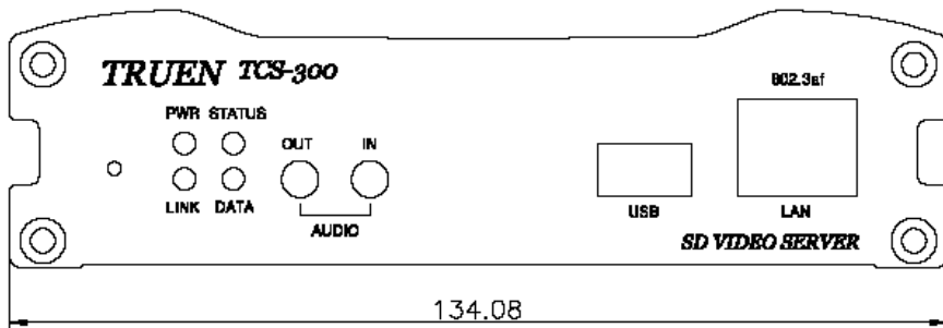
前面
