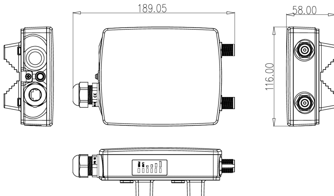
<寸法図> DLB 2
