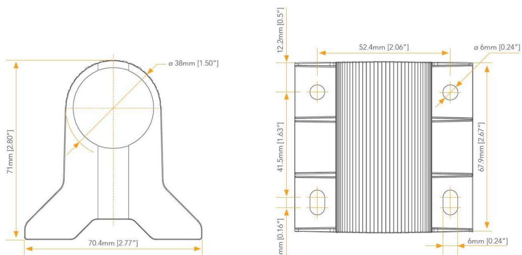
寸法図
