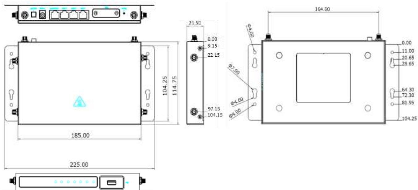
＜寸法図＞ HW5G-3200 本体
