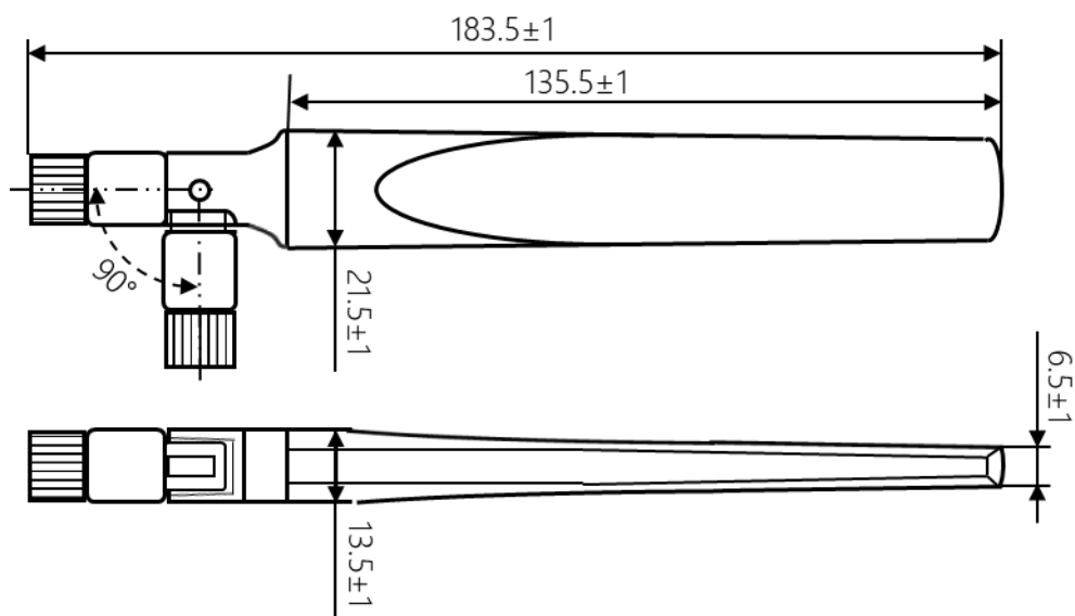
＜寸法図＞ 5G/LTE アンテナ
