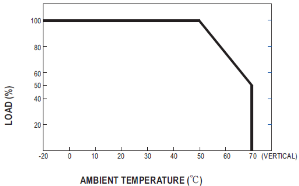
※ディレーティングカーブ
