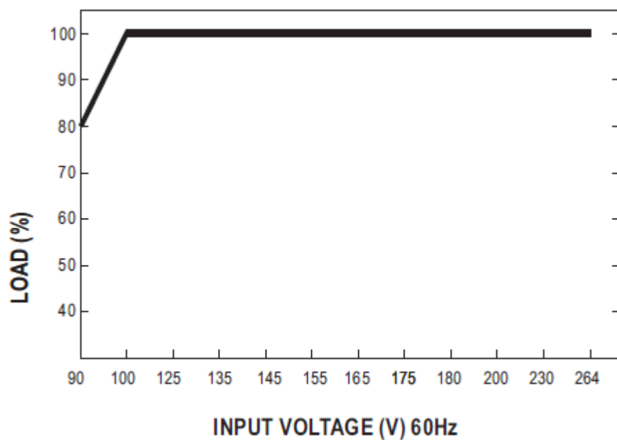
※出力に対する入力電圧
