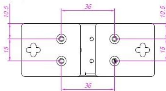
ウォールマウント金具
