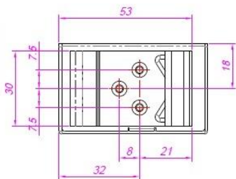
DINレールマウント金具
