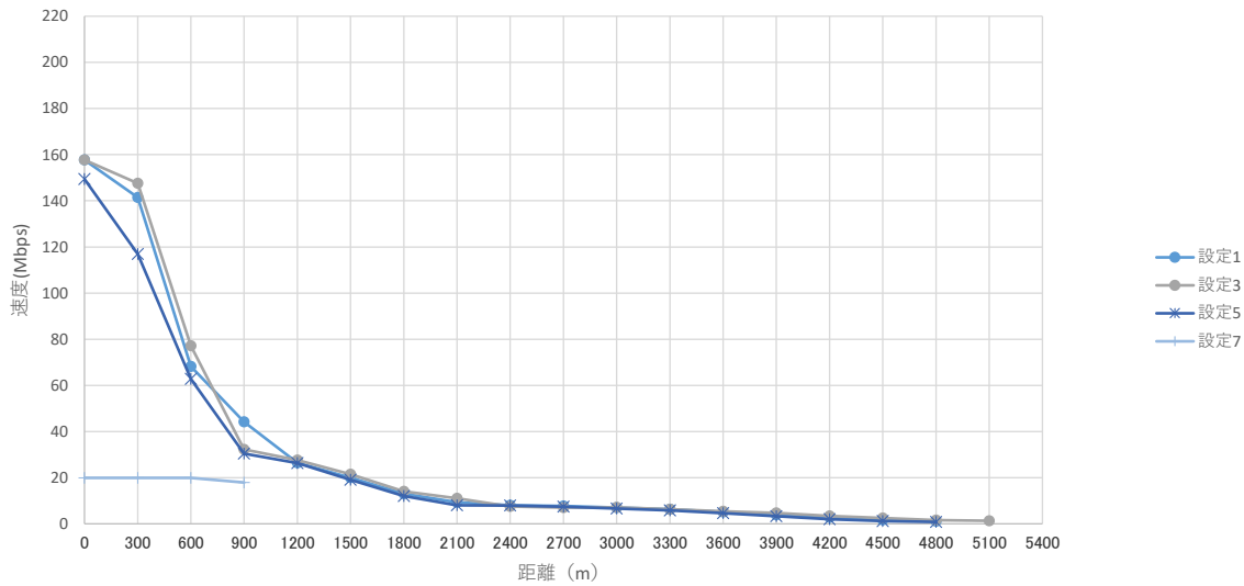
ABiLINX 1002(i)_同期 (Sync) 設定_Down速度比較表
