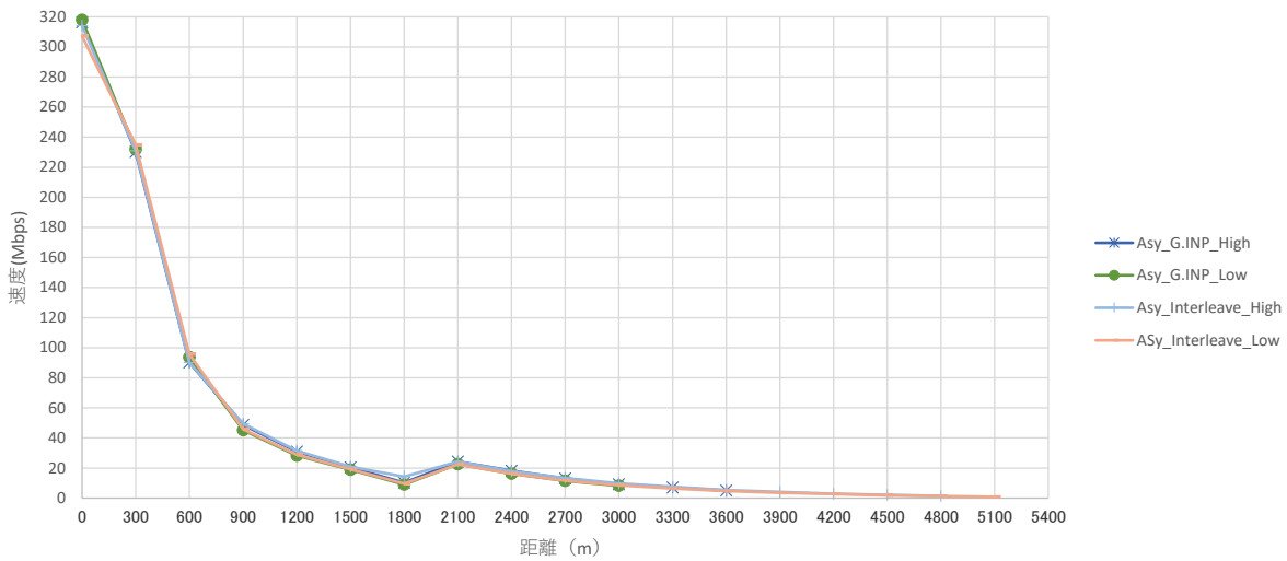
ABiLINX 1003(i)_非同期 (Async) 設定_Down速度比較表
