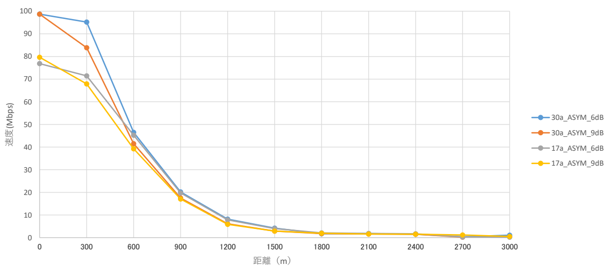
ABiLINX 1001(i)_非同期 (Async) 設定_UP速度比較表
