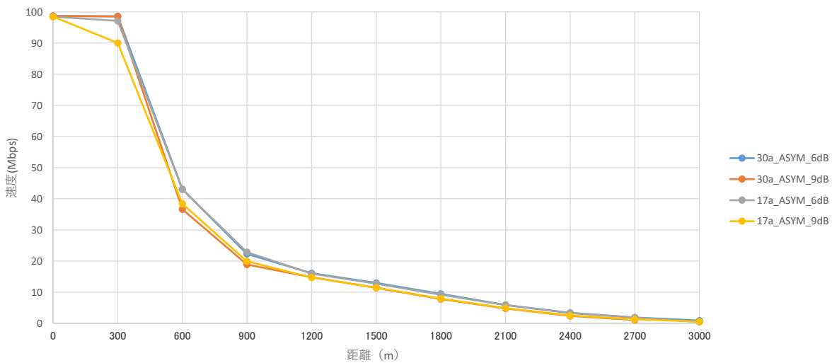
ABiLINX 1001(i)_非同期 (Async) 設定_Down速度比較表
