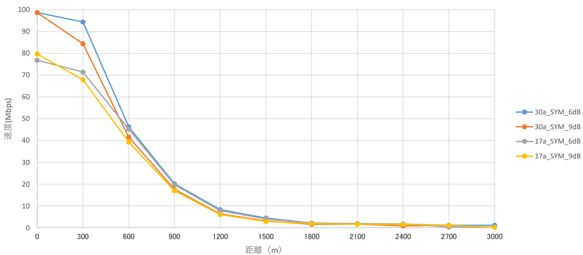
ABiLINX 1001(i)_同期 (Sync) 設定_UP速度比較表
