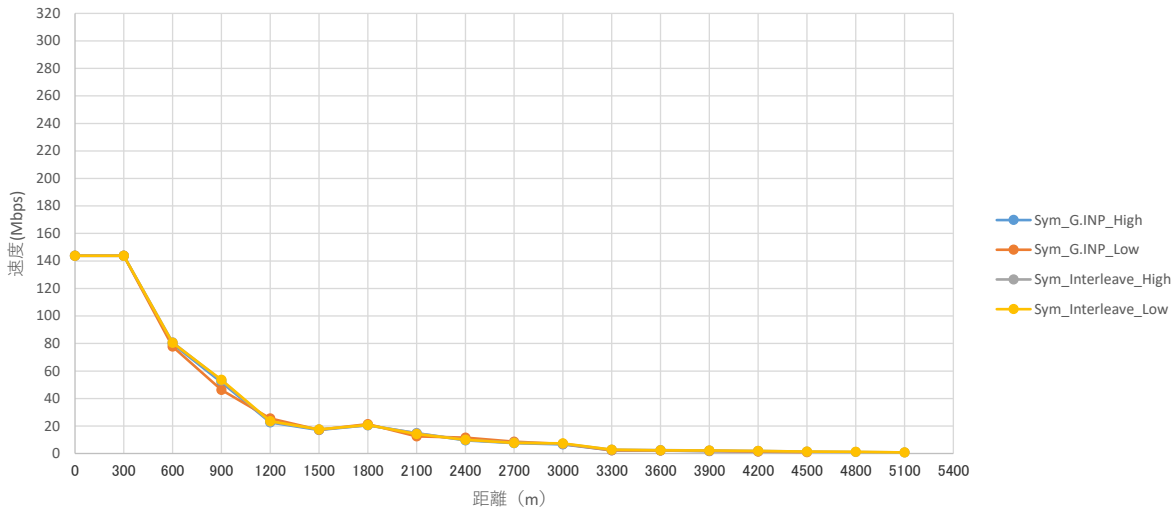
ABiLINX 1003(i)_同期 (Sync) 設定_Down速度比較表
