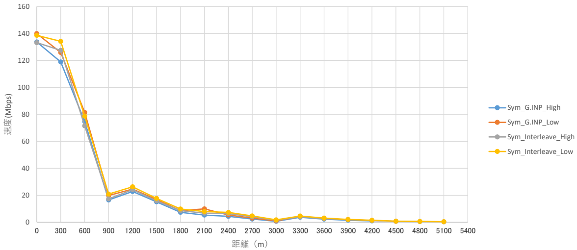
ABiLINX 1003(i)_同期 (Sync) 設定_UP速度比較表
