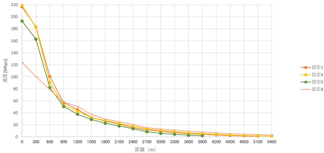
ABiLINX 1002(i)_非同期 (Async) 設定_Down速度比較表
