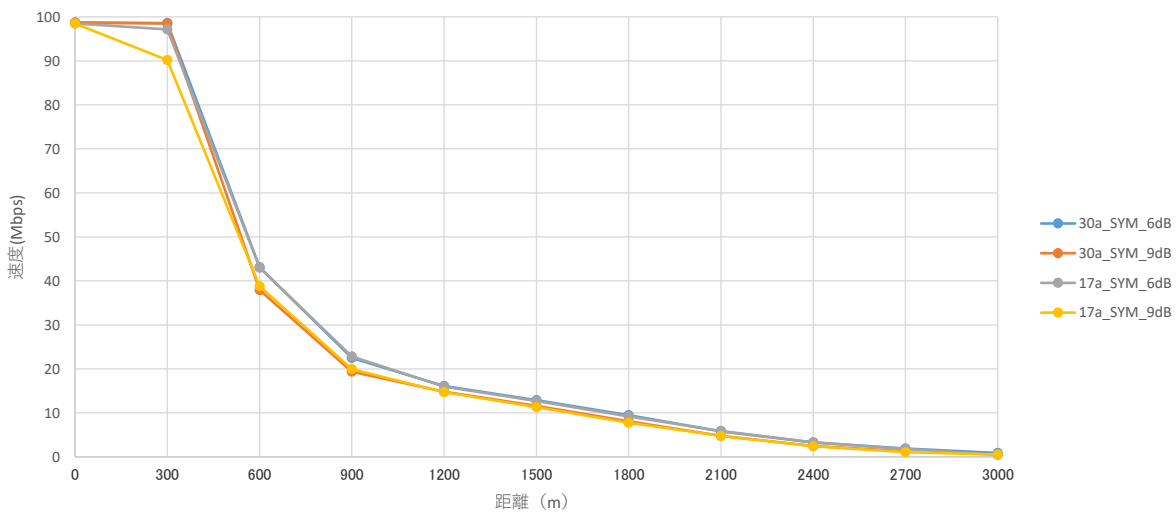
ABiLINX 1001(i)_同期 (Sync) 設定_Down速度比較表
