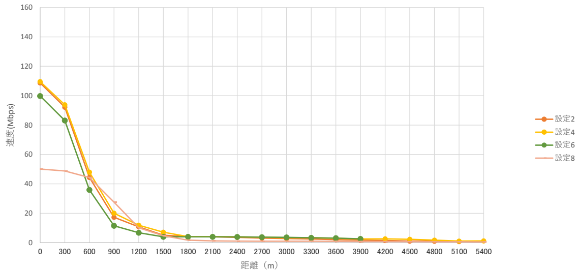
ABiLINX 1001(i)_非同期 (Async) 設定_UP速度比較表
