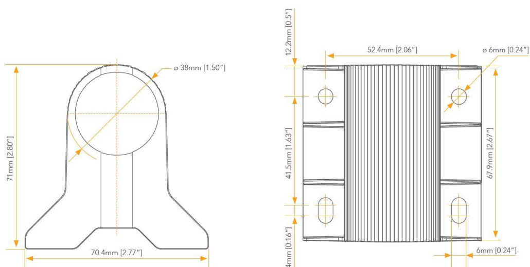
寸法図
