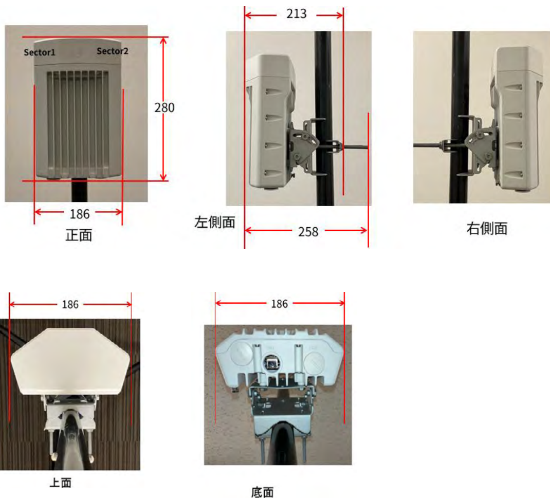
V5000 本体+標準タイプチルト付きブラケット 外観
