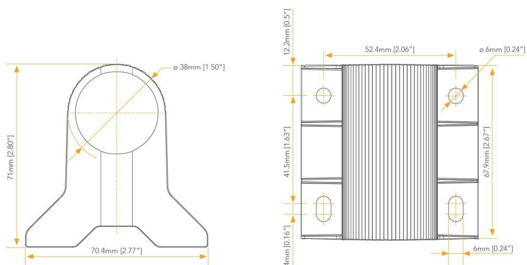
寸法図
